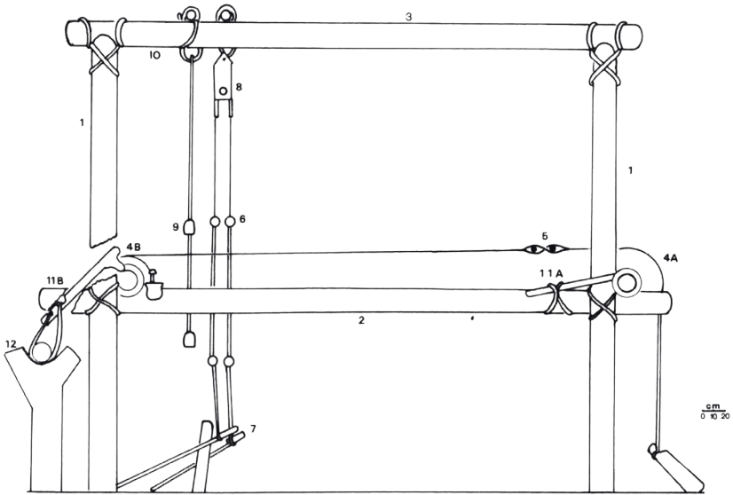
Figura 1: Los componentes del telar: (1) Horcones. (2) Largueros laterales. (3) Cumbreras. (4A) "Julio" trasero. (4B) "Julio" delatentero. (5) "Verdas" o guía-hilos para el cruce de los hilos de la Urdimbre. (6) Lizos. (7) Pedales o "pisones". (8) "Quijada" o polea bascular los lizos. (9) Peine. (Suspensión del peine. (11A) "Garbato". (11B) Garabato. (12) Banco del tejedor.
